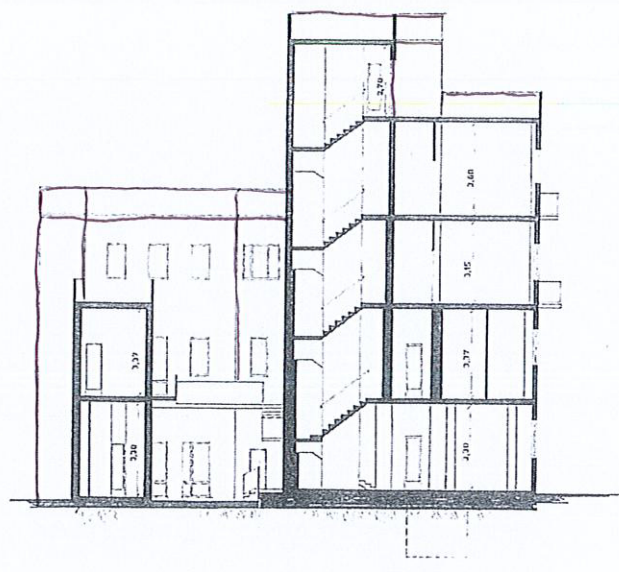
SEZIONE A-A
